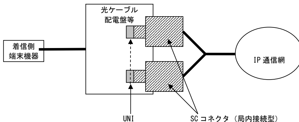
図 12-4 FastEthernetタイプのインタフェース規定点
