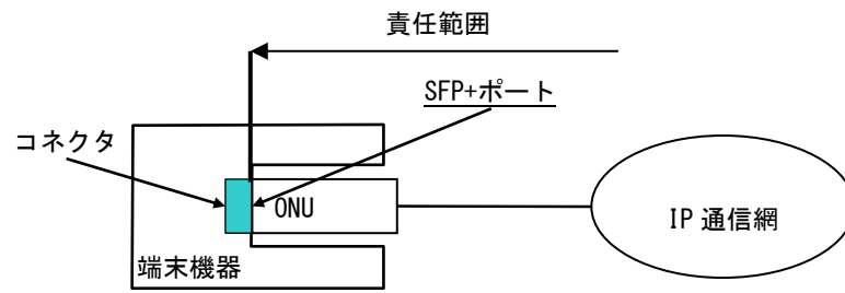
図 4-5 施工・保守上の責任範囲
