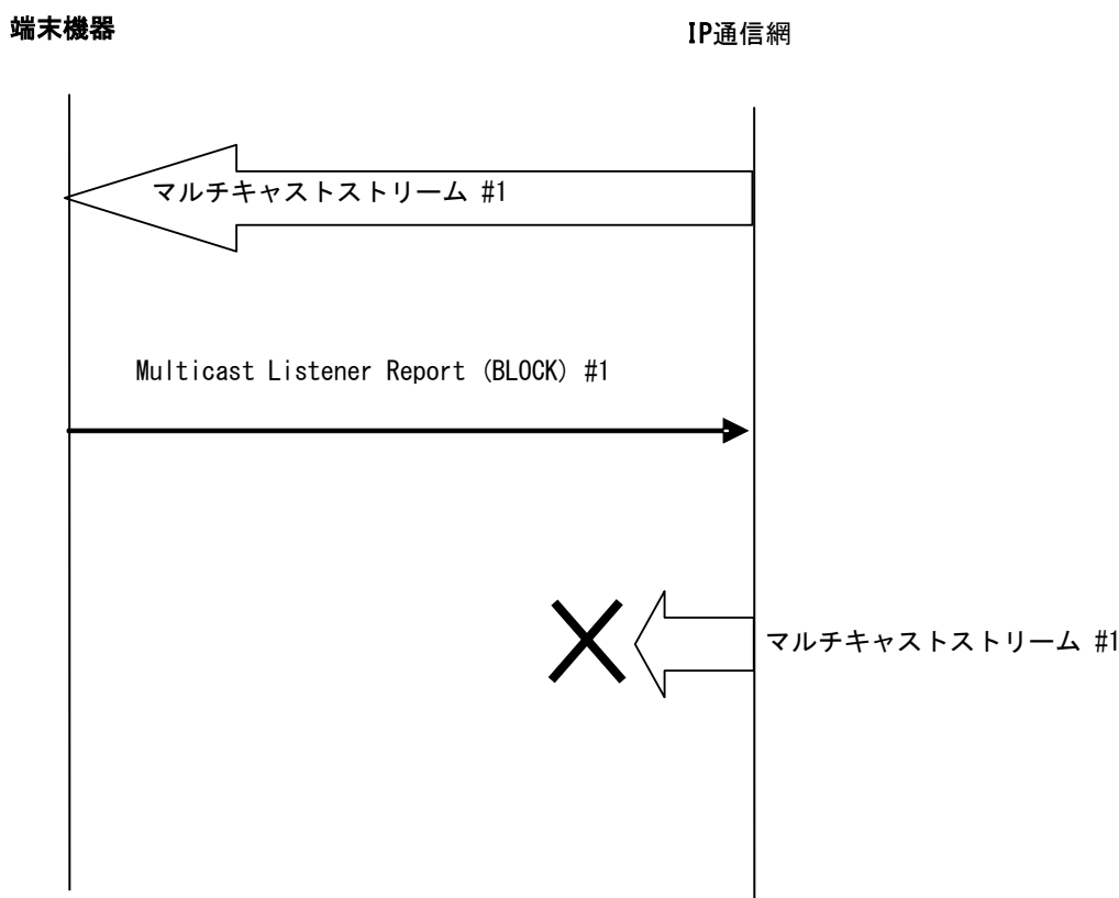
図 5-6 マルチキャスト受信停止シーケンス例
