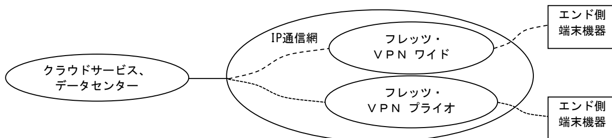
図 23-1 クラウドゲートウェイ クロスコネクの基本構成
