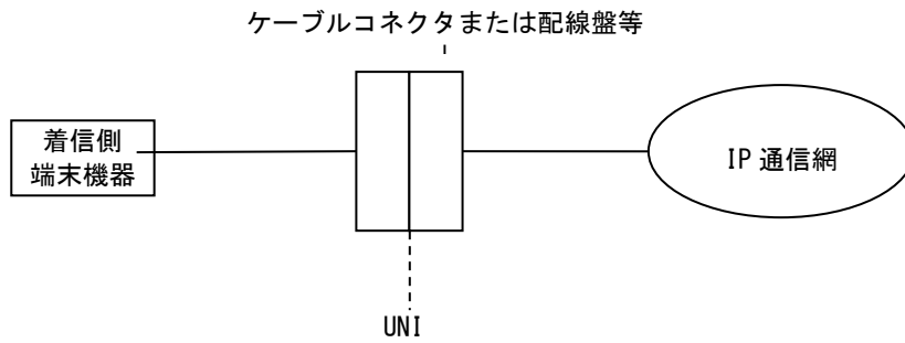
図 17-6 収容エリア内接続タイプのインタフェース規定点
