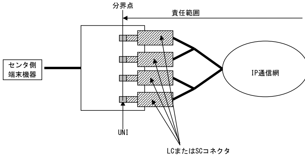
図 23-7 本サービスにおける施工・保守上の責任範囲分界点
