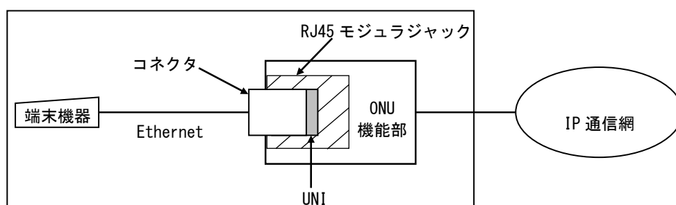
図 11-1 インターフェース規定点
