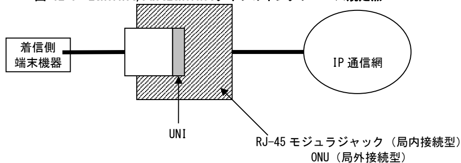
図 12-3 Ethernet/FastEthernetタイプのインタフェース規定点
