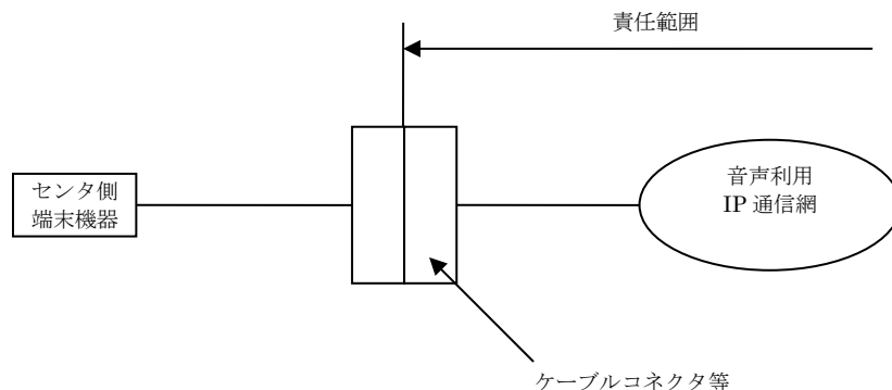
図 2-5-1：ひかり電話ナンバーゲートにおける施工・保守上の責任範囲
